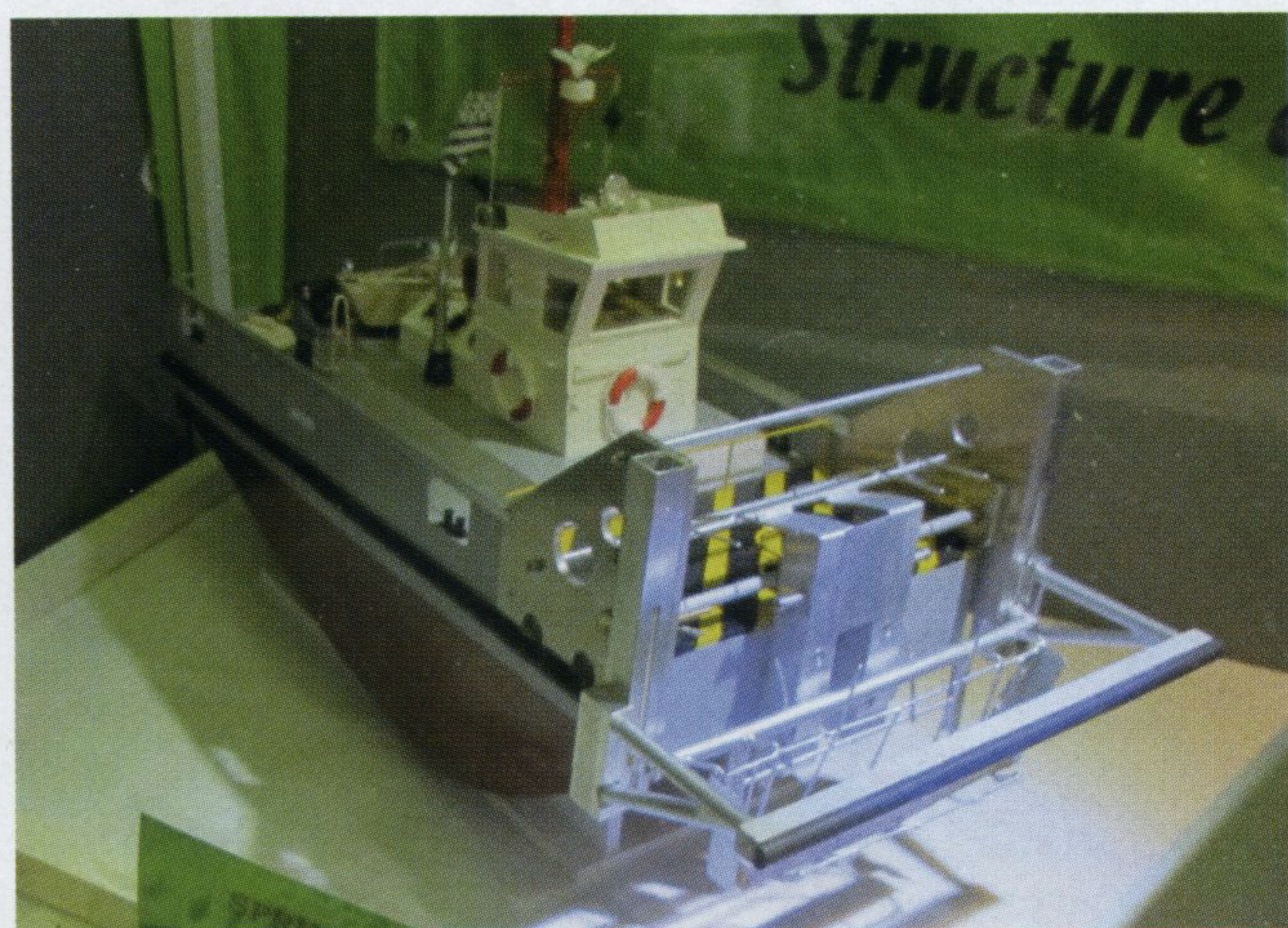
Le Springer ramasseur d'objet de Marc CHARPENTIER.
